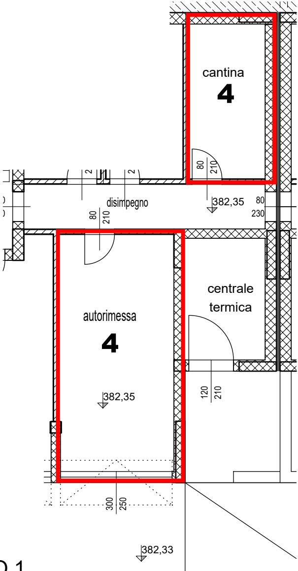
AUTORIMESSA 4 E CANTINA 4 PIANO SEMINTERRATO
